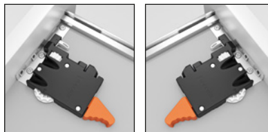
Para clips de fijación AFCGXX3B Derecha e izquierda
